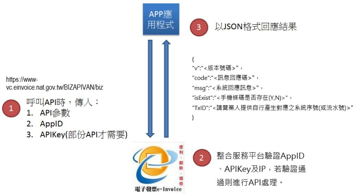
圖 1、電子發票營業人應用 API 使用流程
