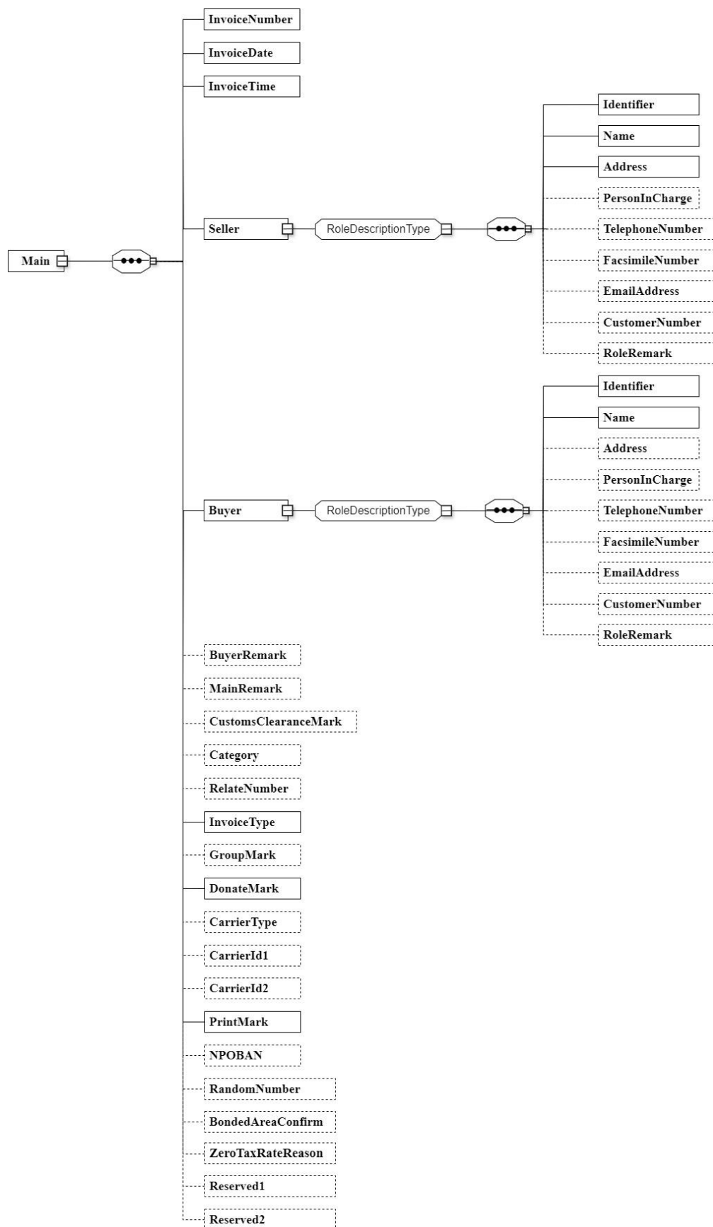
圖 15-3、Invoice/Main 訊息結構圖
