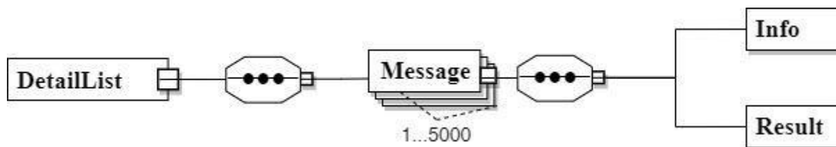
圖 27-4、SummaryResult /DetailList 訊息結構圖
