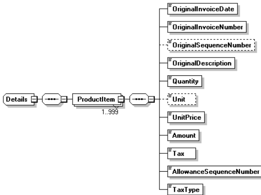
圖45：Allowance/Details 訊息結構圖
