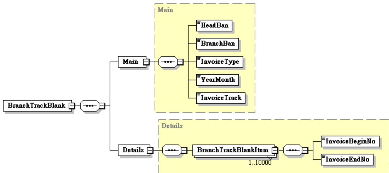
圖 52：E0402 訊息結構圖
