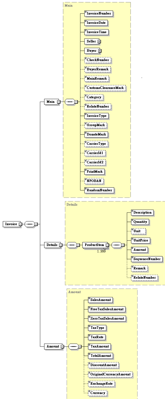
圖35：C0401訊息結構圖
