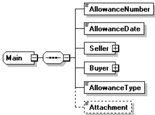
圖12：Allowance/Main訊息結構圖
