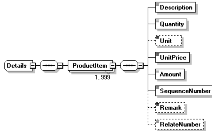
圖7：Invoice/Detail 訊息結構圖
