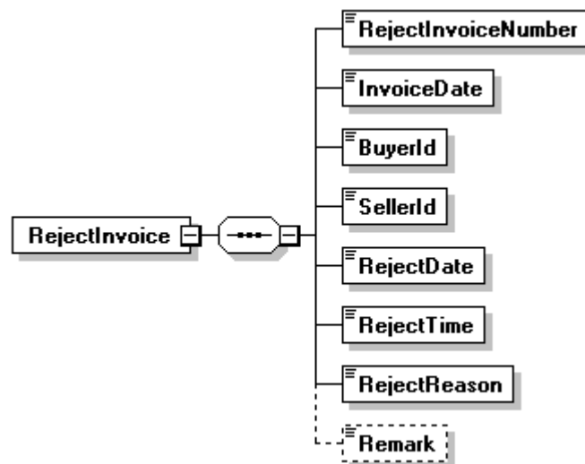
圖34：A0601訊息結構圖
