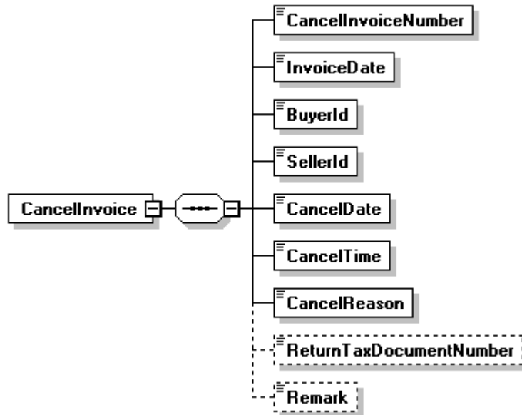
圖 32：A0501 訊息結構圖
