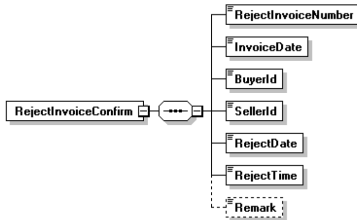
圖21：A0302訊息結構圖
