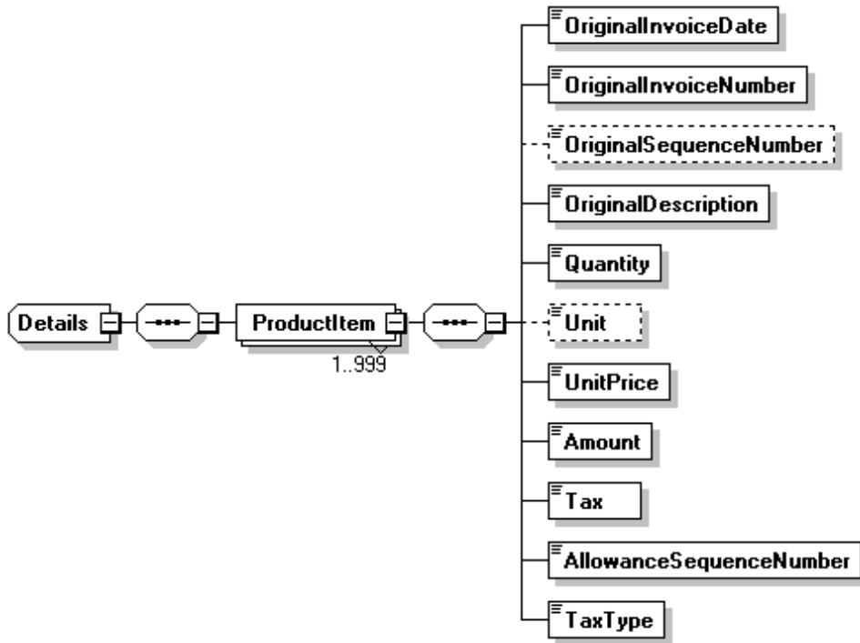
圖 13：Allowance/Details 訊息結構圖
