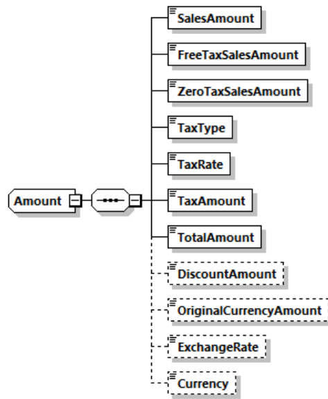
圖39：Invoice/Amount 訊息結構圖
