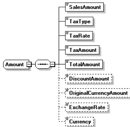
圖8：Invoice/Amount 訊息結構圖
