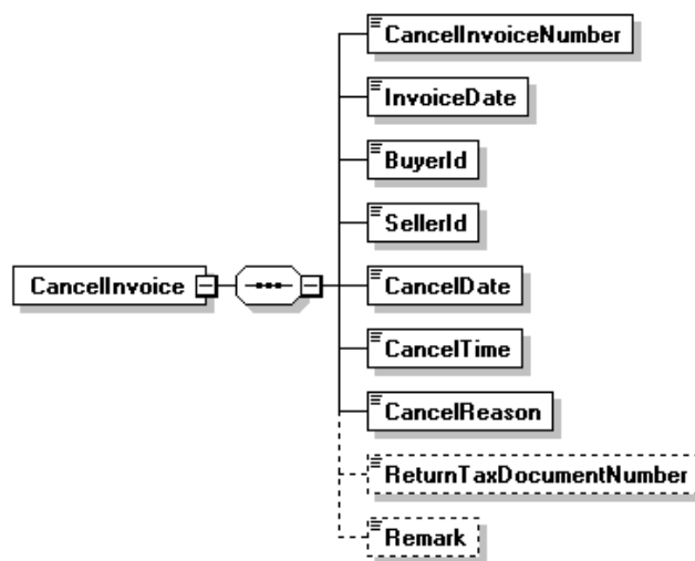
圖40：C0501訊息結構圖
