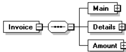
圖23：Invoice訊息結構圖
