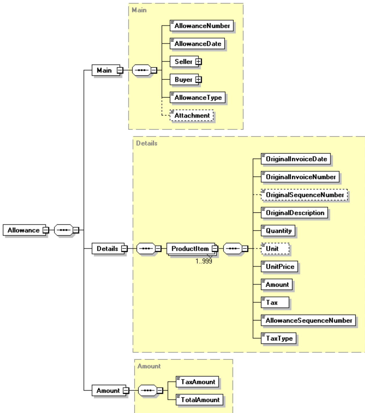
圖 10：B0101 訊息結構圖
