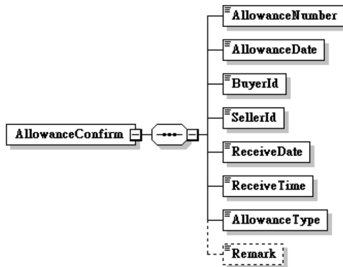
圖 15：B0102 訊息結構圖
