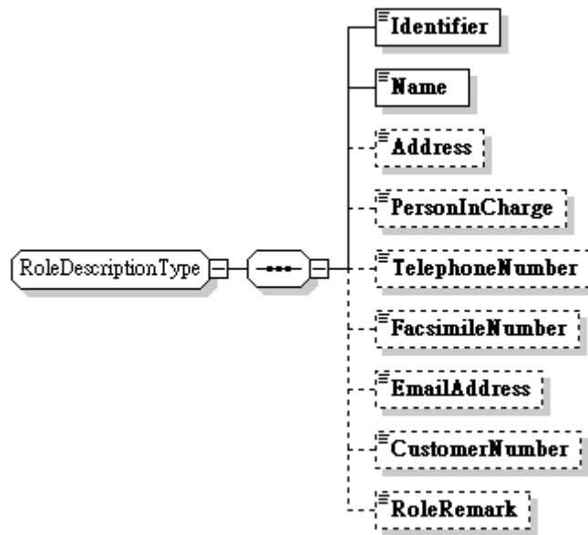
圖3：RoleDescriptionType 訊息結構圖
