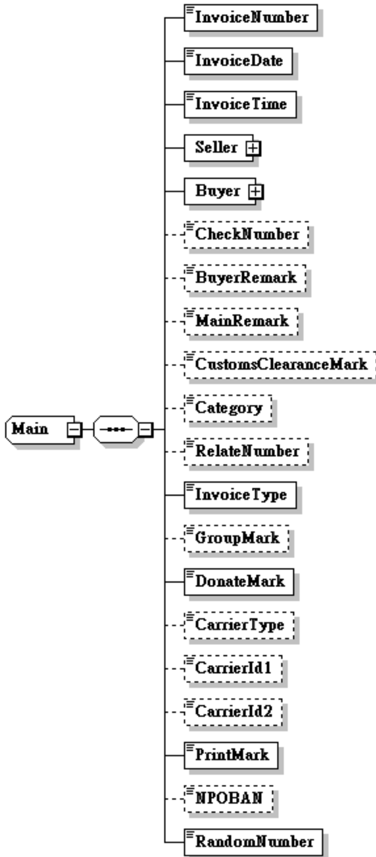
圖37：Invoice/Main訊息結構圖
