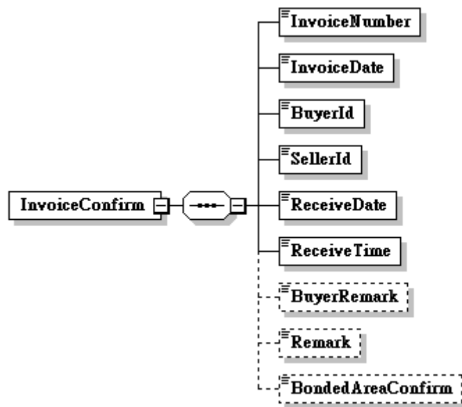
圖9：A0102訊息結構圖
