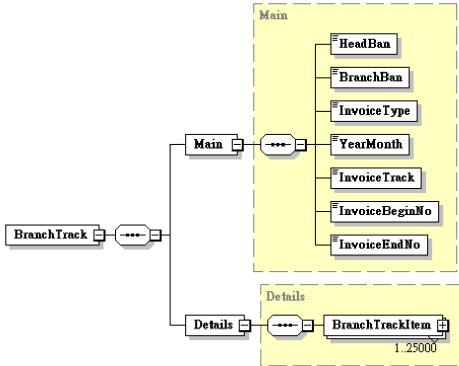
圖48：E0401訊息結構圖
