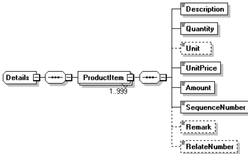
圖 38：Invoice/Detail 訊息結構圖
