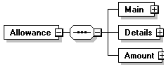
圖11：Allowance訊息結構圖
