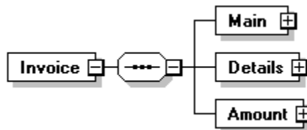
圖5：Invoice訊息結構圖
