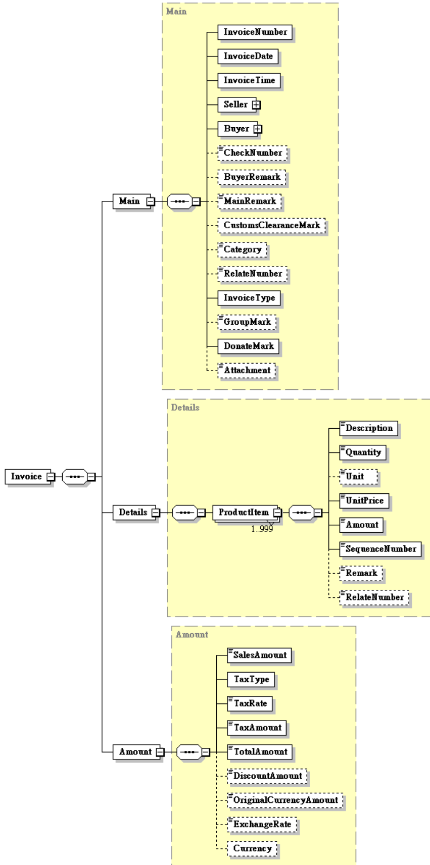
圖4：A0101 訊息結構圖
