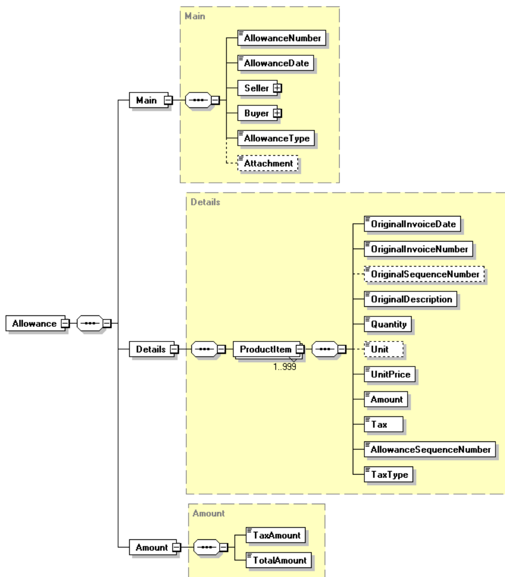
圖42：D0401訊息結構圖
