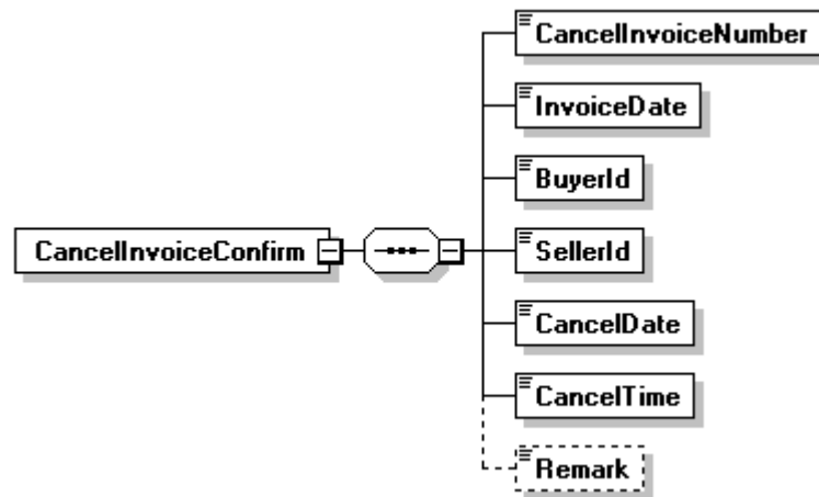
圖17：A0202訊息結構圖
