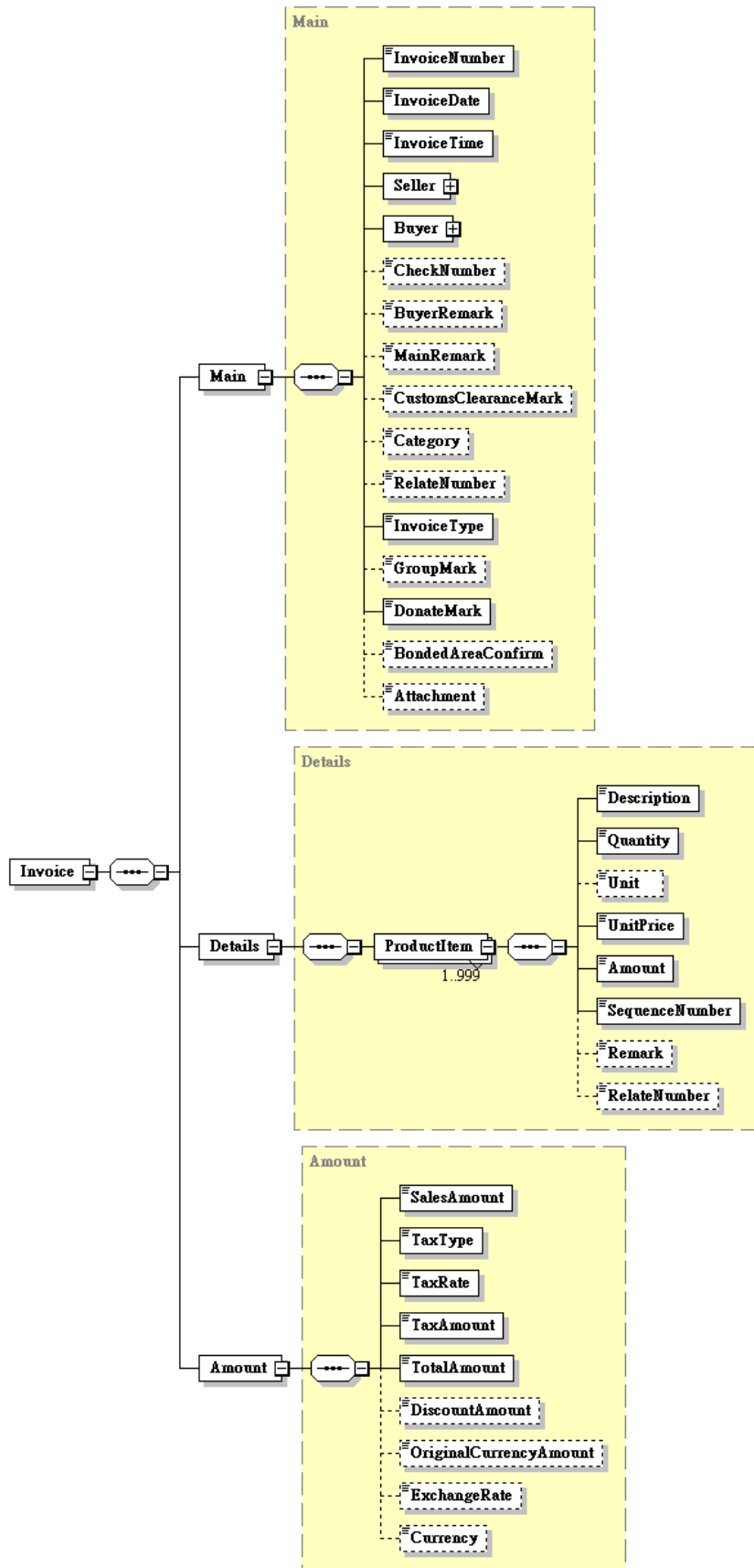
圖22：A0401訊息結構圖
