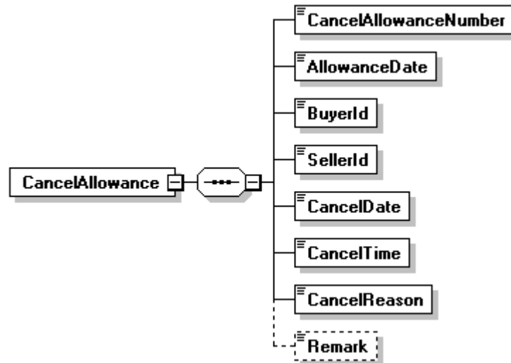
圖18：B0201 訊息結構圖
