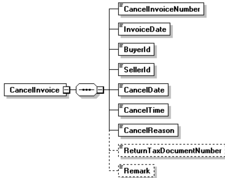
圖 16：A0201 訊息結構圖
