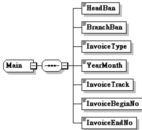
圖50：BranchTrack /Main訊息結構圖
