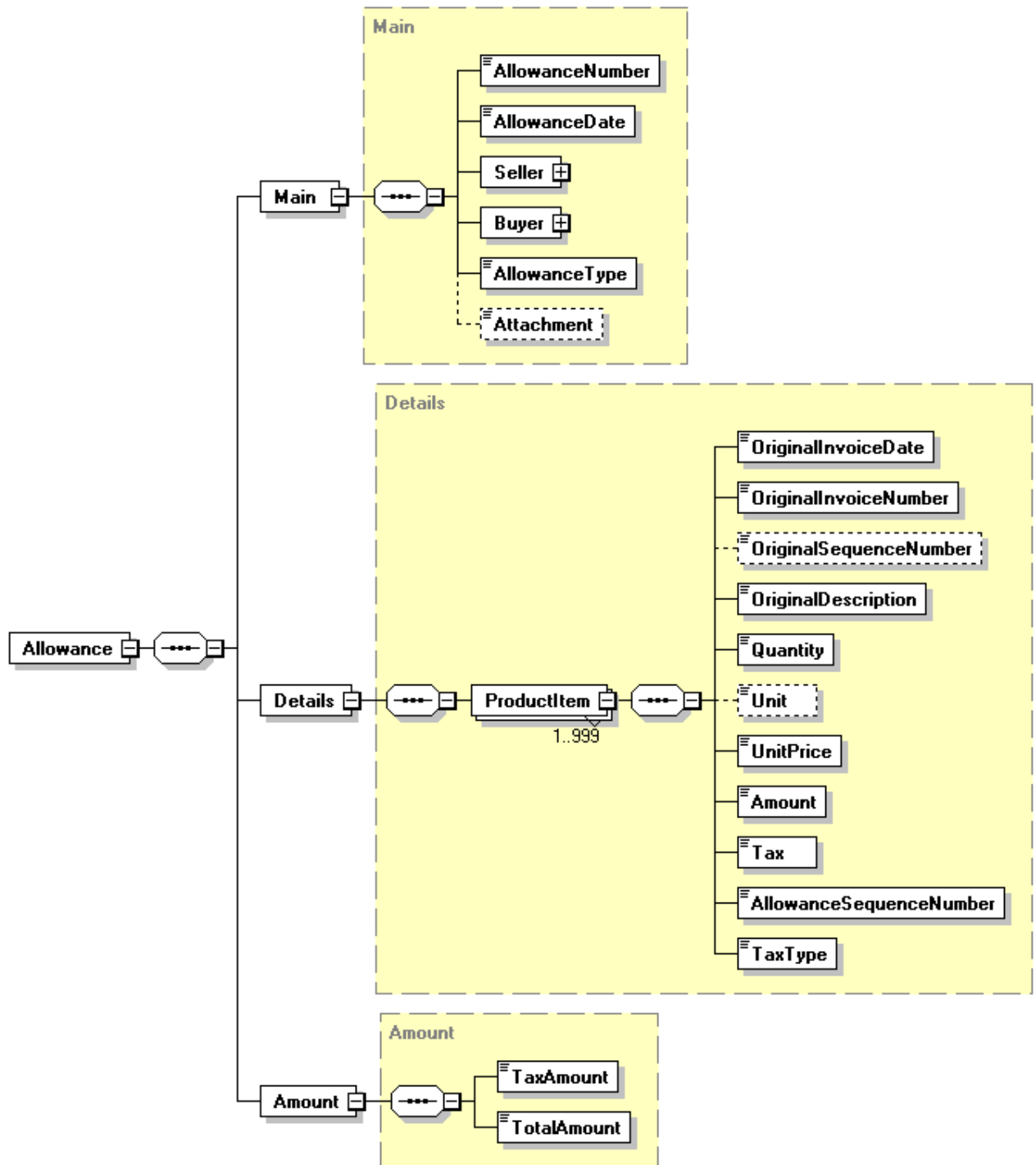
圖27：B0401 訊息結構圖
