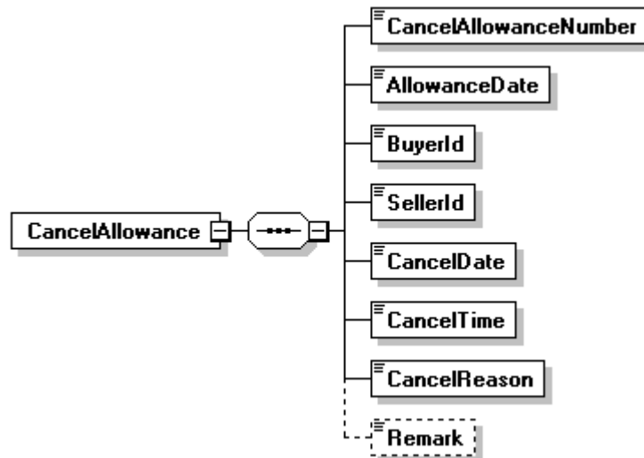
圖33：B0501訊息結構圖
