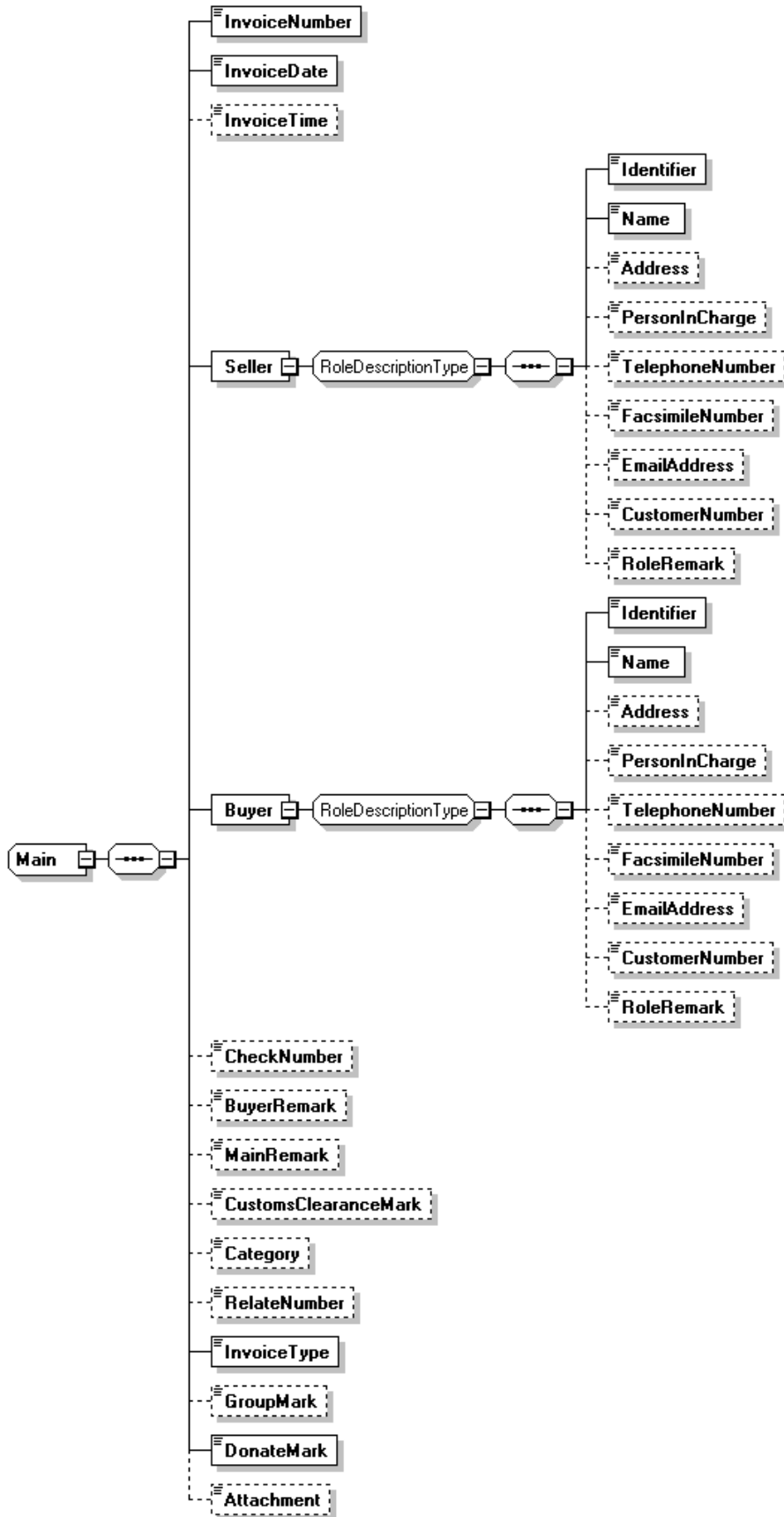
圖6：Invoice/Main訊息結構圖
