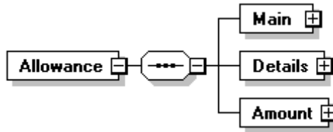
圖28：Allowance訊息結構圖
