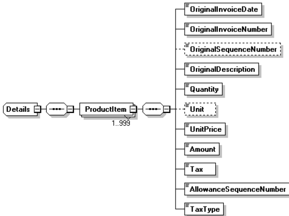
圖30：Allowance/Details訊息結構圖
