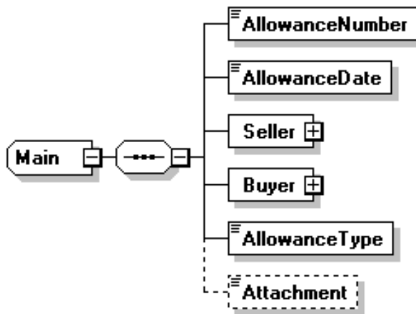
圖29：Allowance/Main訊息結構圖
