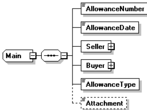
圖44：Allowance/Main訊息結構圖
