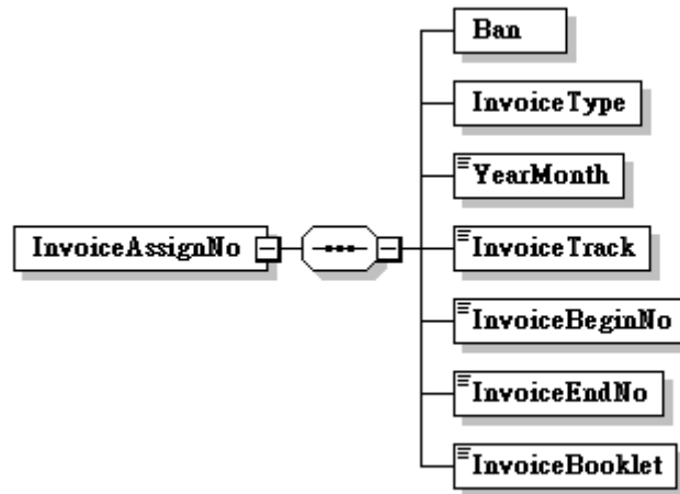
圖56：E0501訊息結構圖
