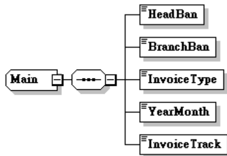
圖54：BranchTrackBlank/Main訊息結構圖
