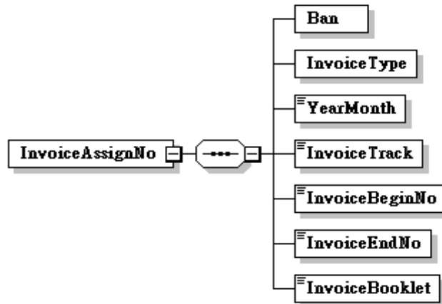
圖57：InvoiceAssignNo訊息結構圖
