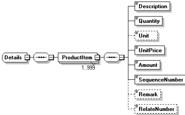
圖25：Invoice/Detail訊息結構圖
