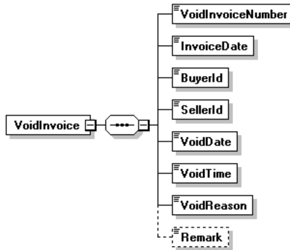
圖41：C0701訊息結構圖
