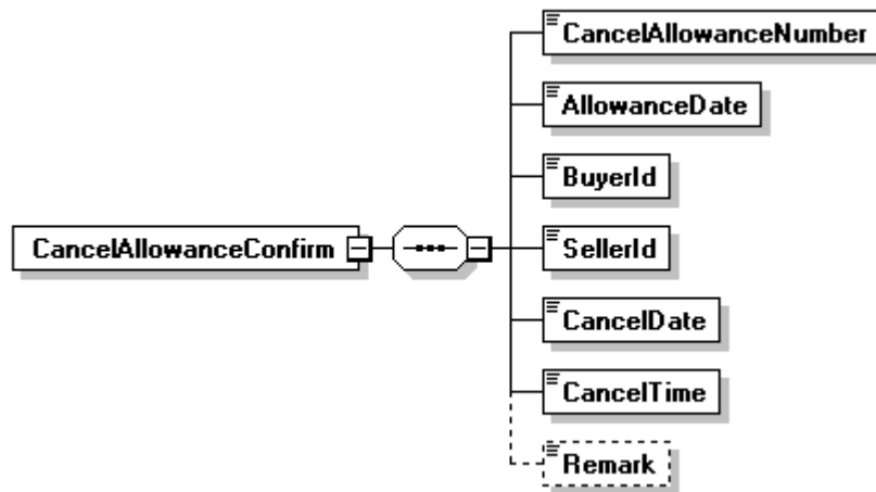
圖 19：B0202 訊息結構圖
