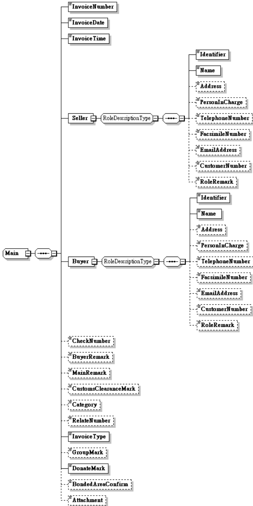
圖24：Invoice/Main訊息結構圖
